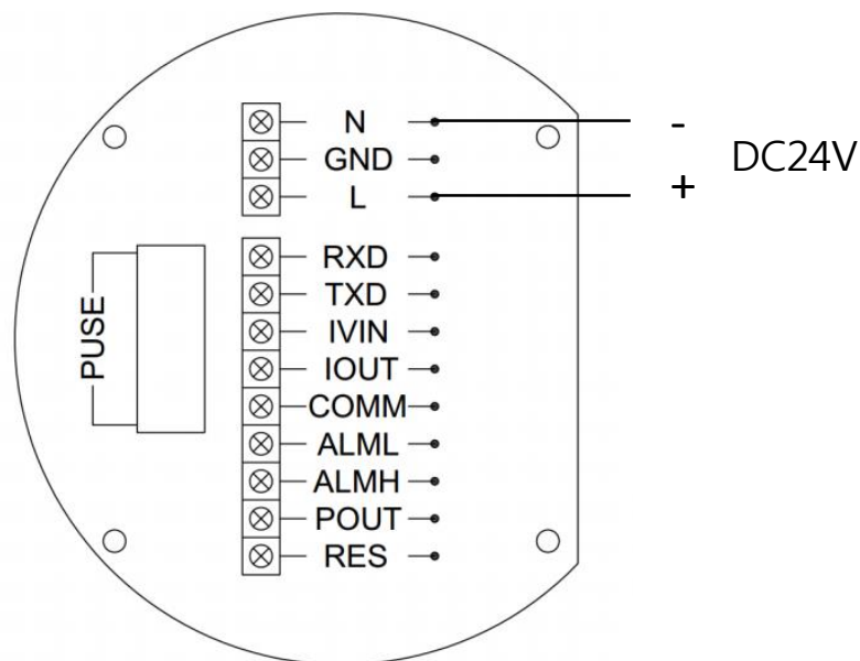
그림.5: 단자대
