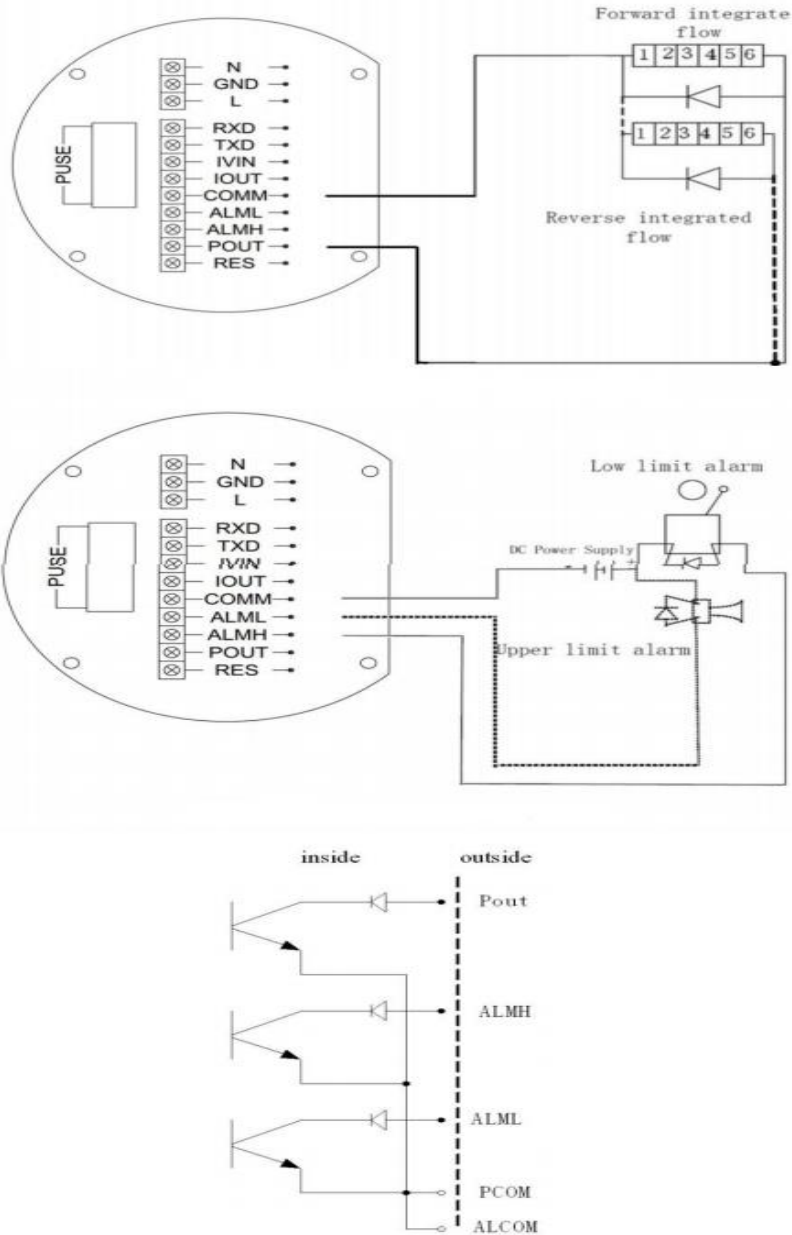
그림.6: 출력 결선도
