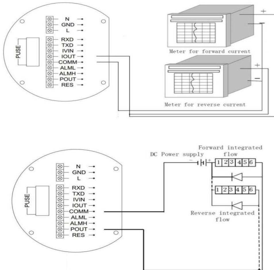
그림.6: 출력결선도
