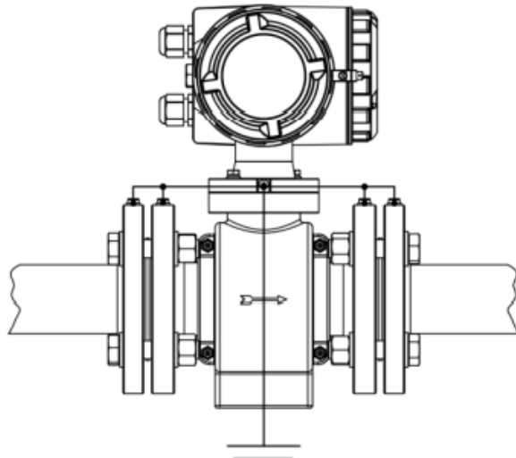
그림 12 : 라이닝 된 파이프에 접지 옵션 또는 접지 전극 없음
